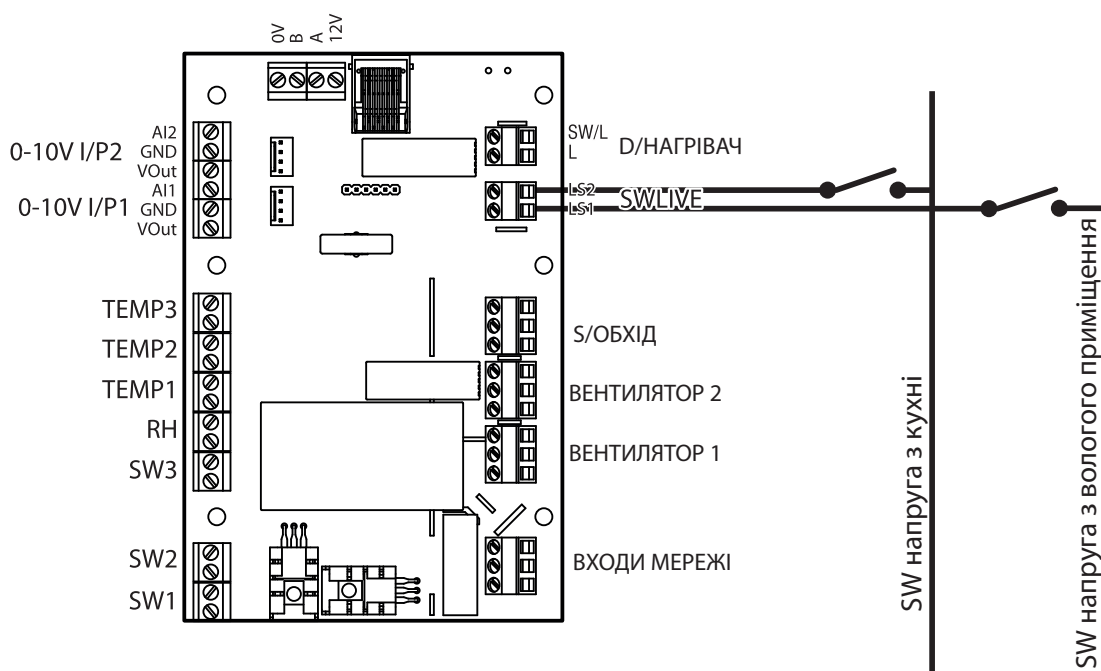
Входи перемикачів ПІД НАПРУГОЮ, поз. ЕЕ163
