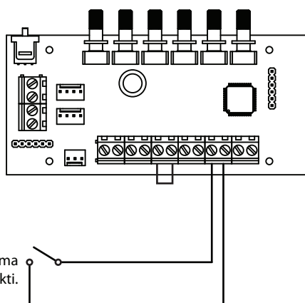
Samazinājuma režīma pārslēgšana un savienojums ref EE177
