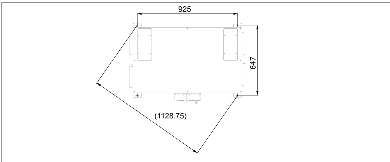
Ubicaciones de fijación H200 y H300
