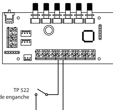
Conexión de interruptor SUMMERboost® ref EE178
