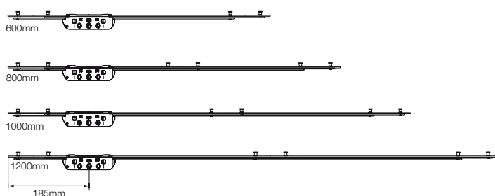
R.A.I.L. Reach Espagnolette dimensions
