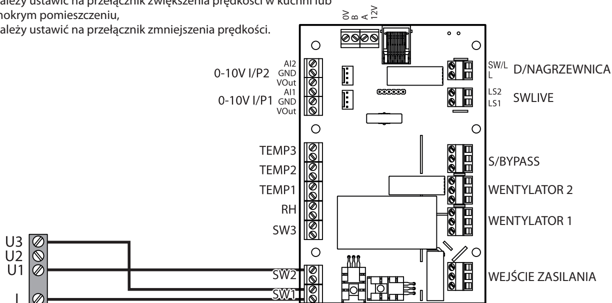
Złącza łącznika pokrętnego trójpozycyjnego, nr ref. EE162
