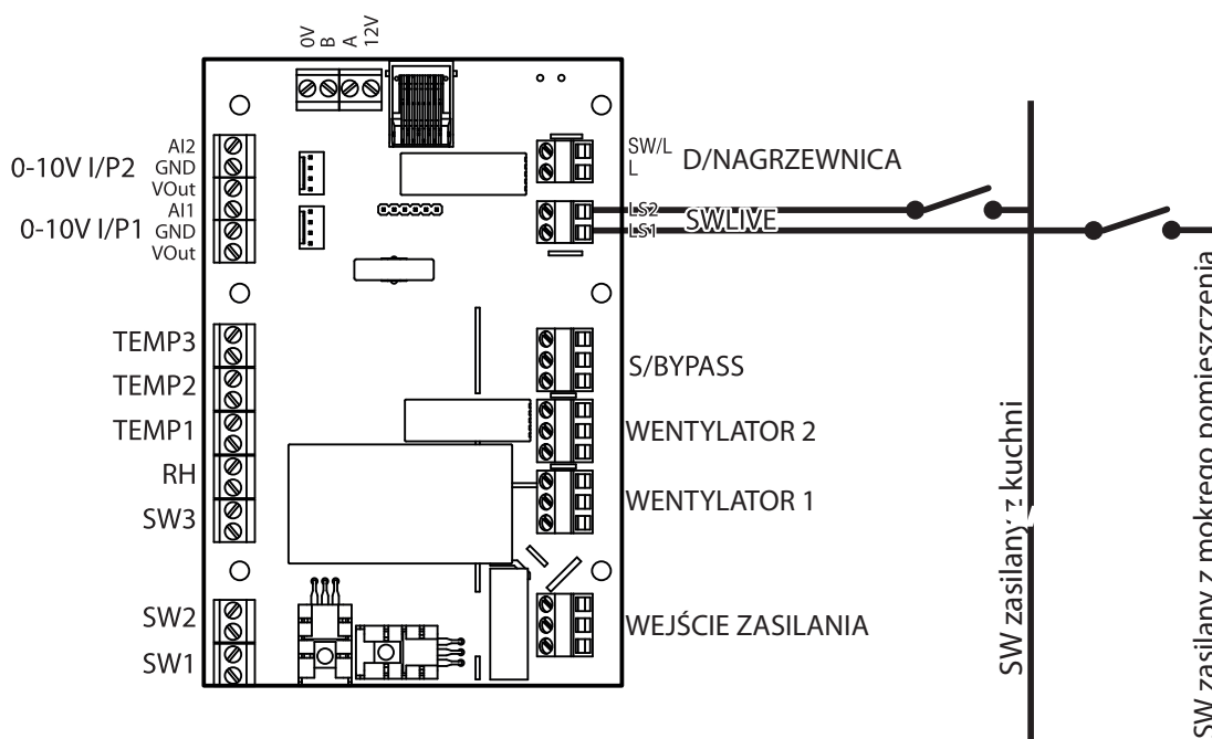
Wejścia przełącznika napięciowego, nr ref. EE163
