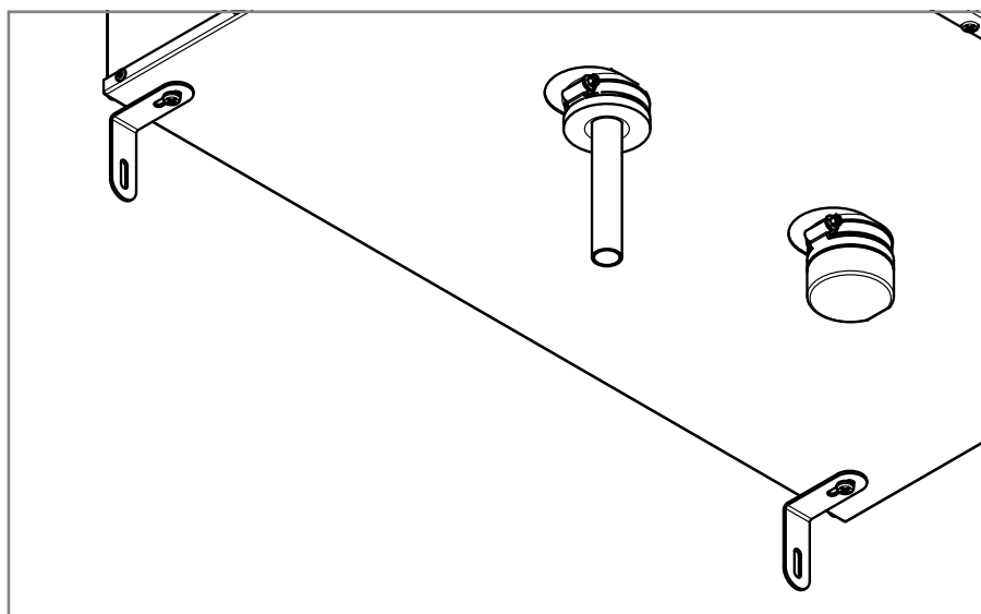
Wspornik bezpieczeństwa
